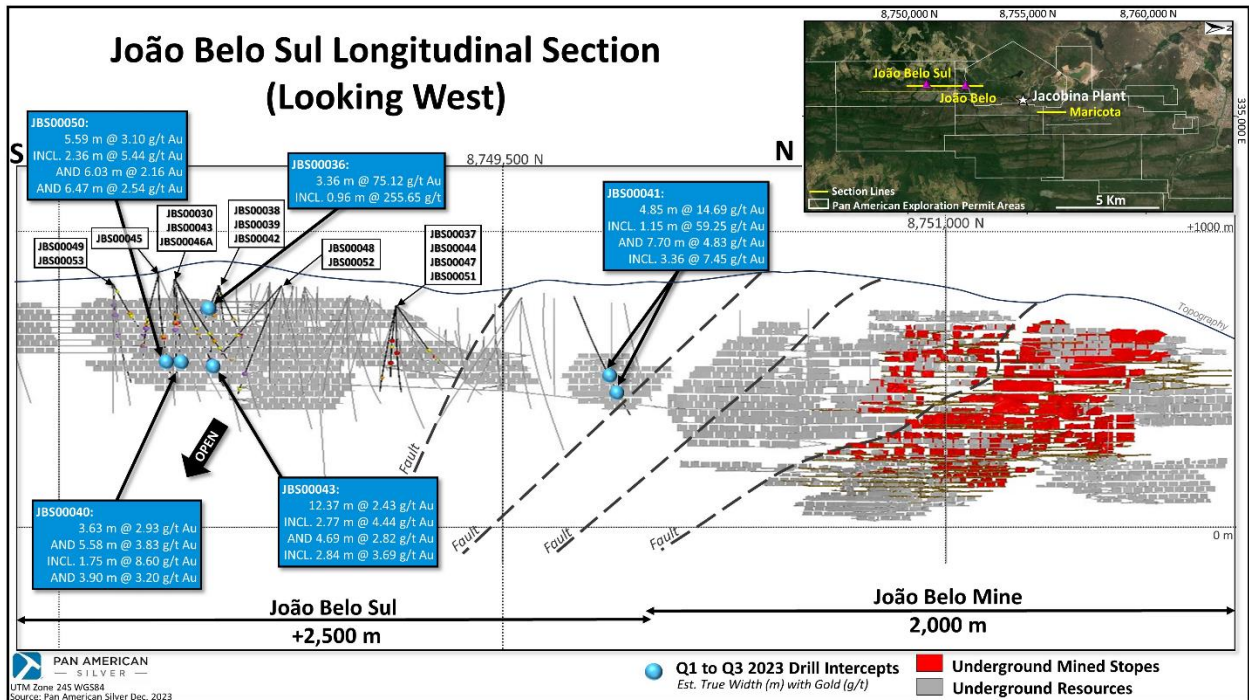
Figure 2. Jacobina - João Belo Sul Long Section
